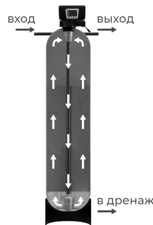
1. Обратная промывка
